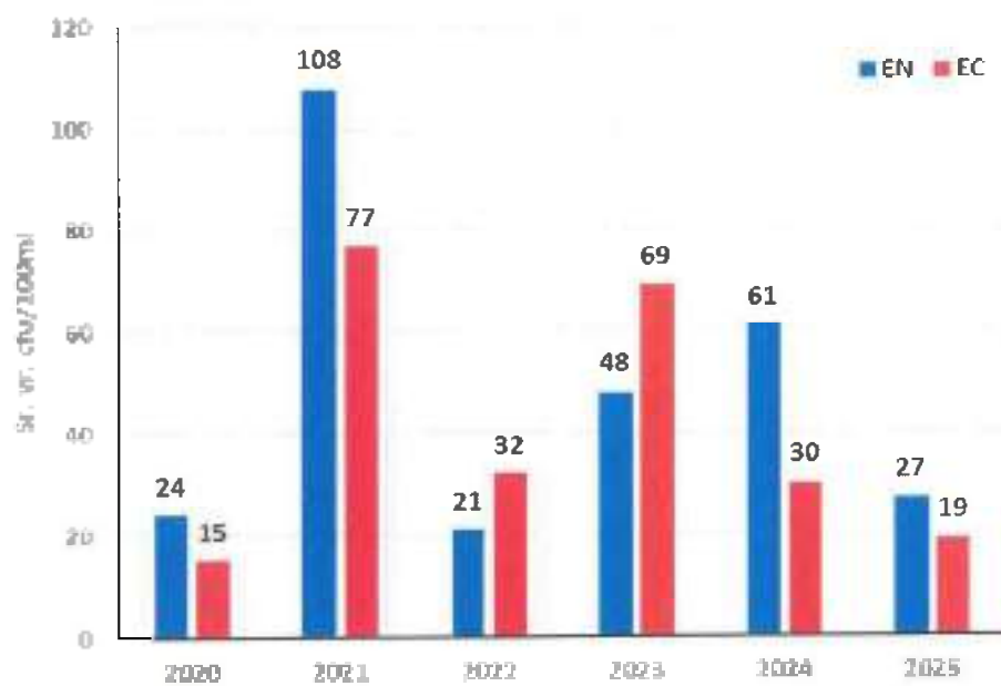
Slika 4. Kretanje koncentracije srednjih vrijednosti ispitivanih mikrobioloških parametara (EN – crjevni enterokoki i EC – Escherichia coli ) u periodu od 2020.-2025. na kupalištu Baier-Čoka
